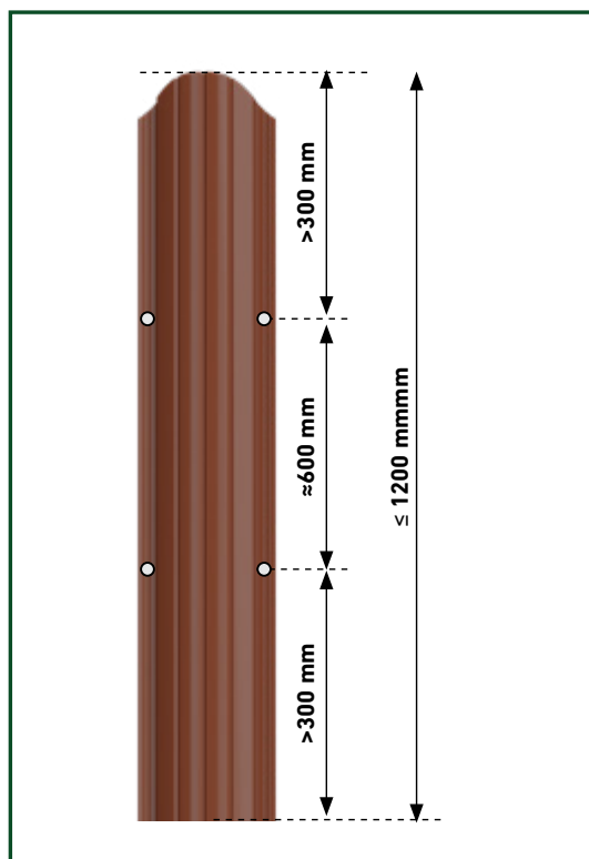
Fig. 1. Pentru șipca cu H \leq 1200 mm, vor fi prinderi cu 4 șuruburi.
