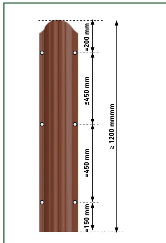
Fig. 2. Pentru șipca cu H \geq 1200 mm sunt recomandate minim 6 șuruburi.
